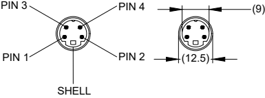
4 PIN MINI DIN MALE MATING FACE
