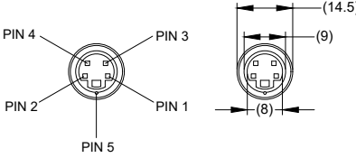
4 PIN MINI DIN FEMALE MATING FACE
